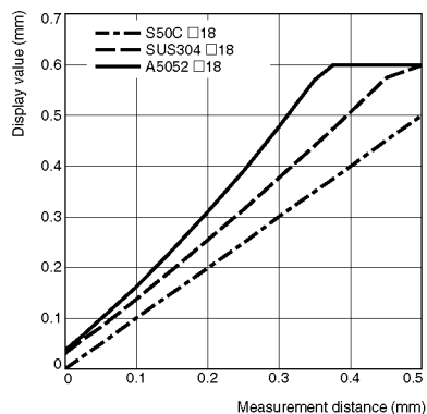
ZX-EM07MT
